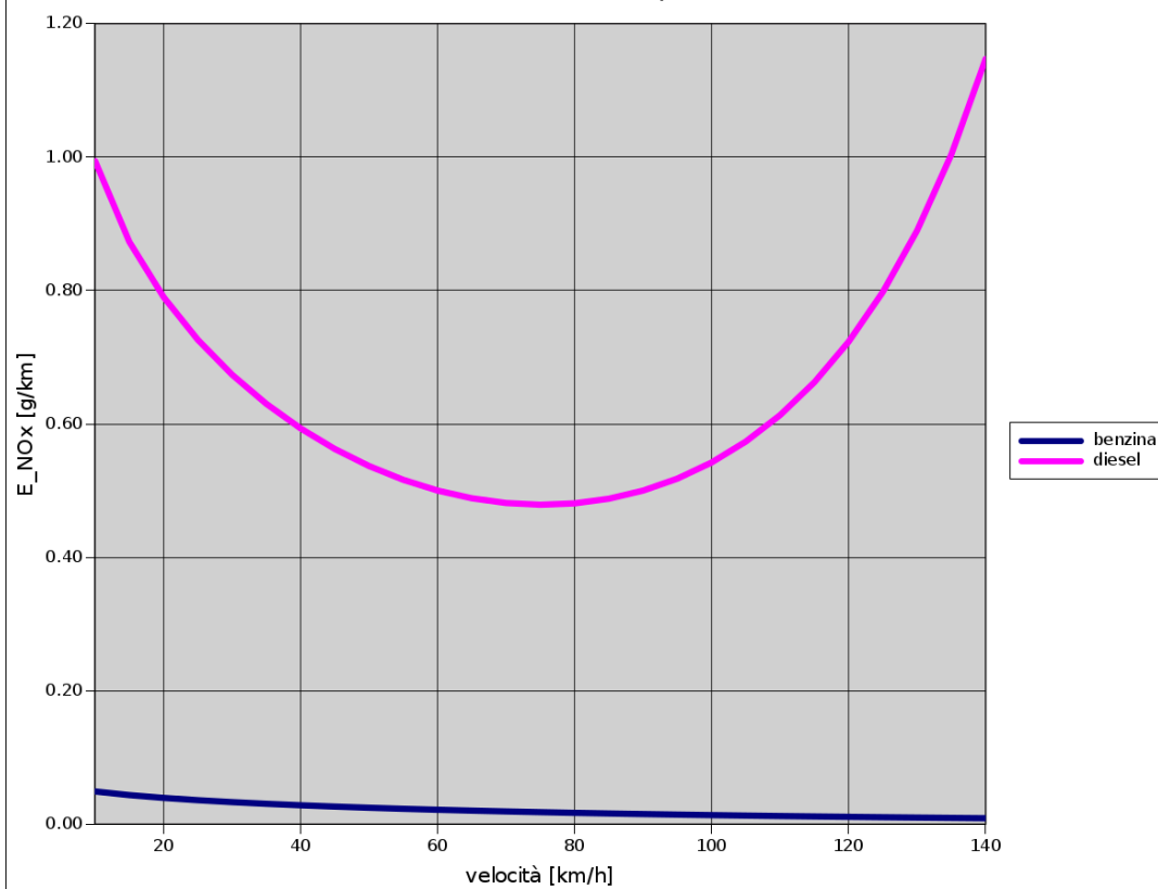
Emissione NOx benzina / diesel Euro 5
